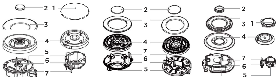
Piezas de los quemadores
